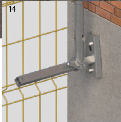
Fassadenhalterung
