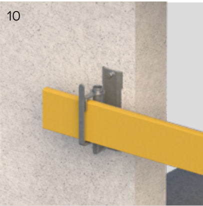
Wandhalterung
