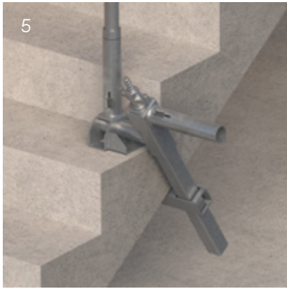
Stufenhalterung
