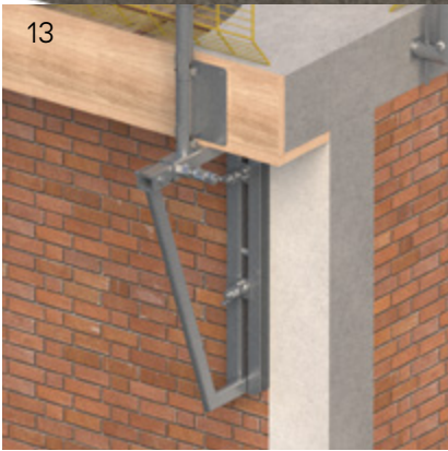
Schalunghalterung
