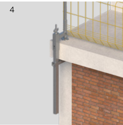
L500/L800 Spannzangenhalterung
