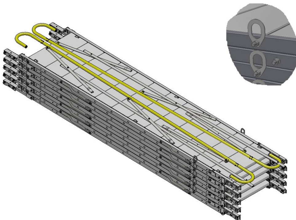
Rys 4. Składowanie schodów
