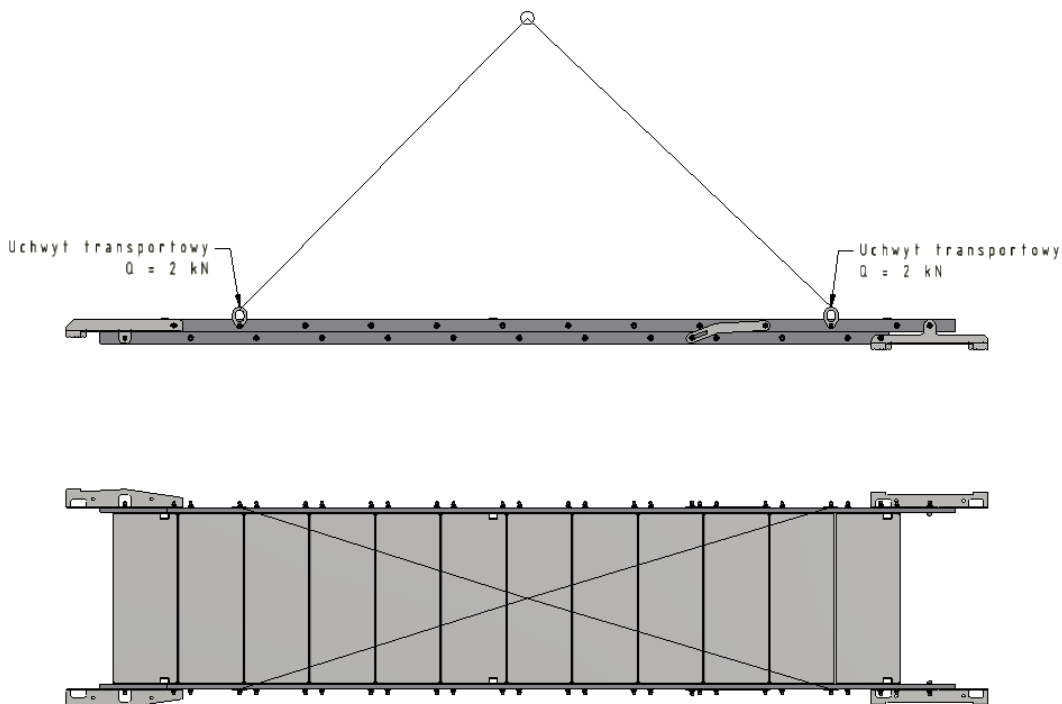
Rys 1. Rysunek schodni
