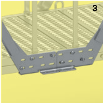
Anschlussstelle Fußgängerüberweg
