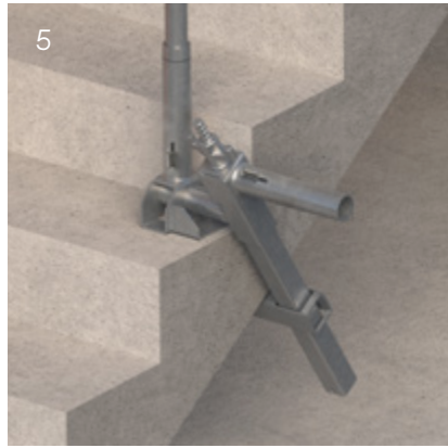
Uchwyt schodowy
