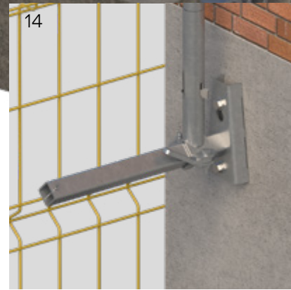
Uchwyt fasadowy
