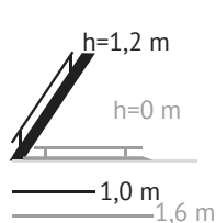
6 Stufen
